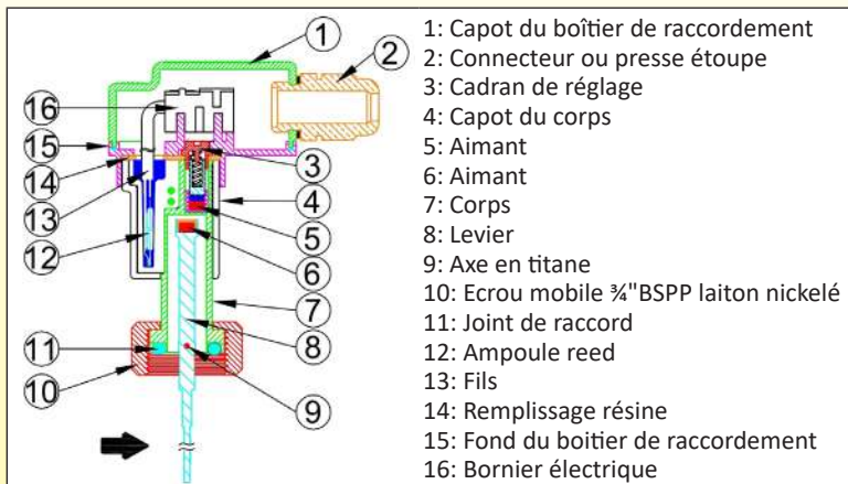
Modèle à deux aimants, mécanisme externe, réglable
