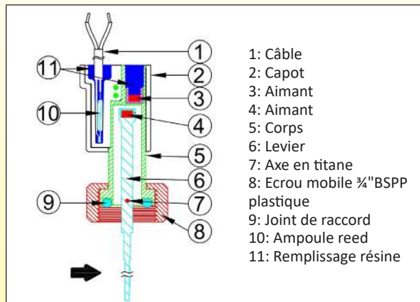
Modèle à deux aimants, mécanisme externe, non réglable
