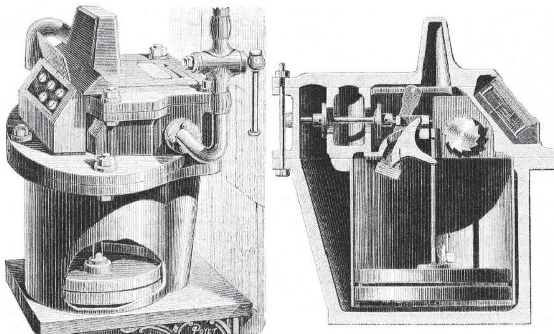
1881, dans les premiers compteurs d'eau de la ville de Paris, la mesure est effectuée par un système à piston (système Jacquet)
